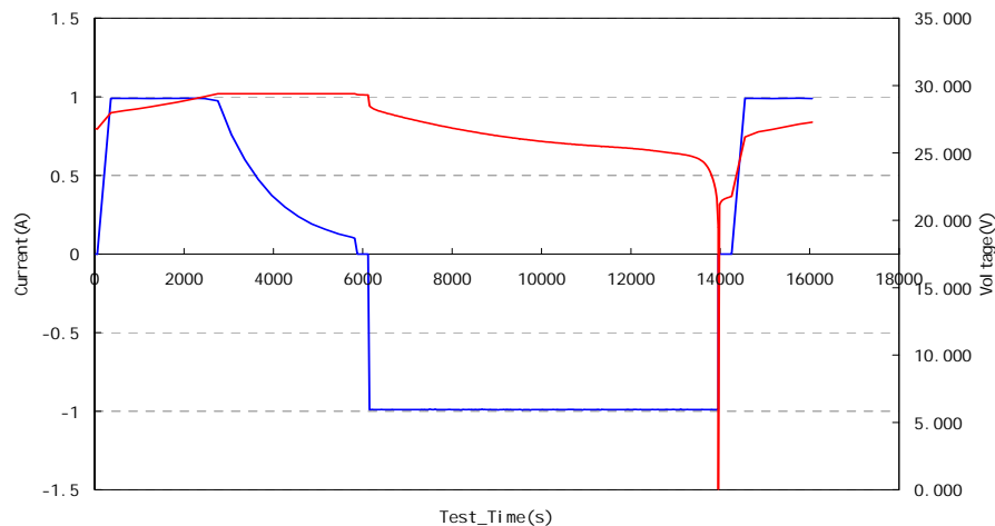
车载电源模块用锂离子电池组充放电曲线
