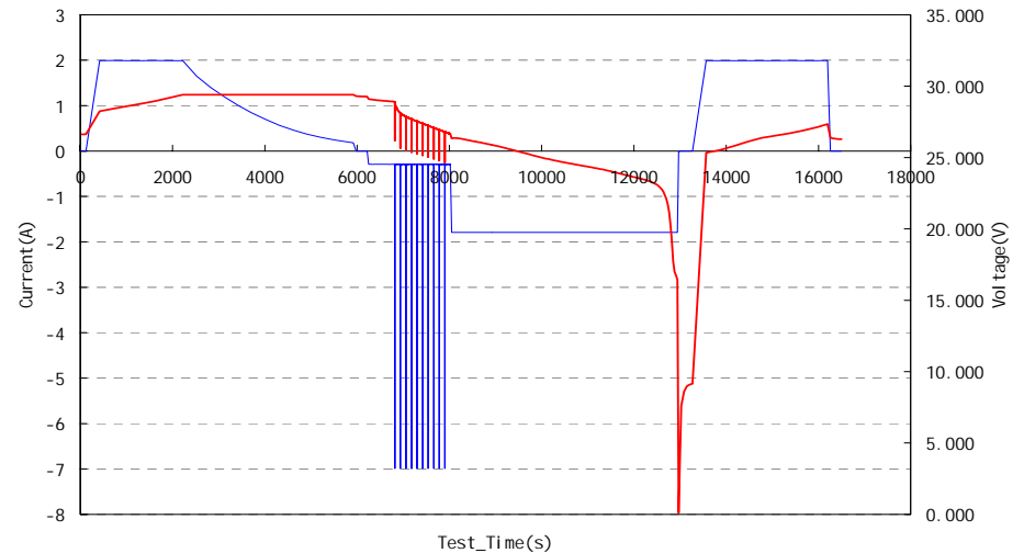
71CR1865-2锂离子电池组充放电曲线
