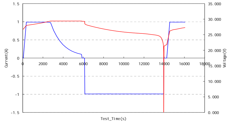
71CR1865( )锂离子电池组充放电曲线
