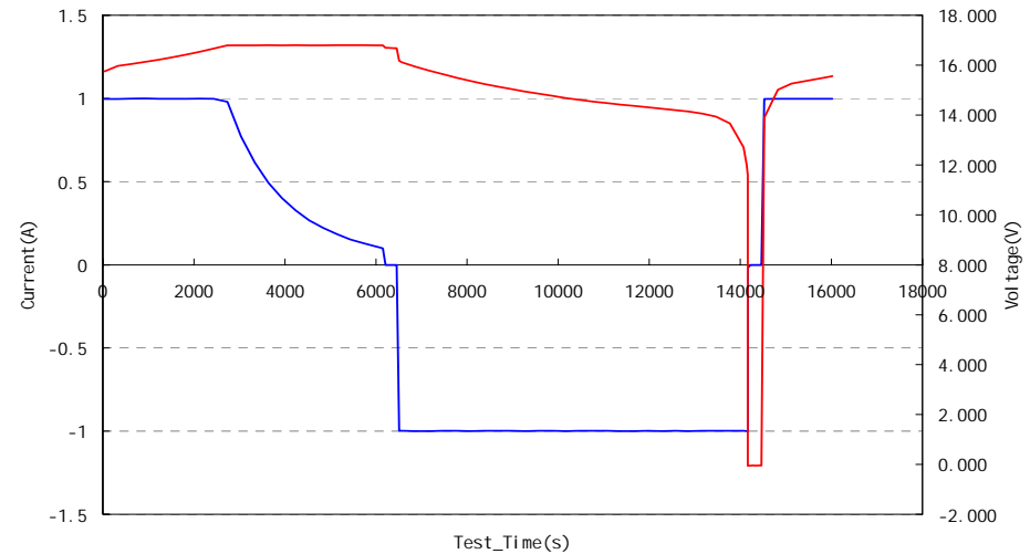
41CR1865锂离子电池组充放电曲线
