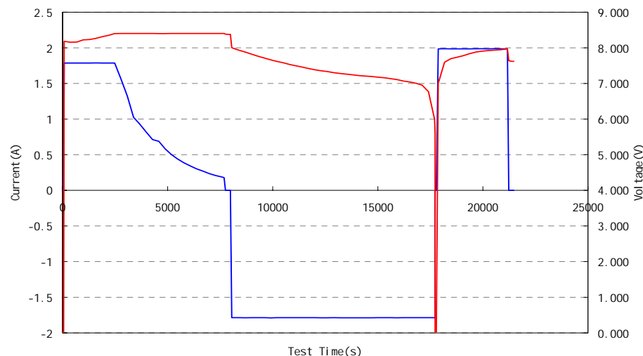
2I CR1865-2锂离子电池组充放电曲线
